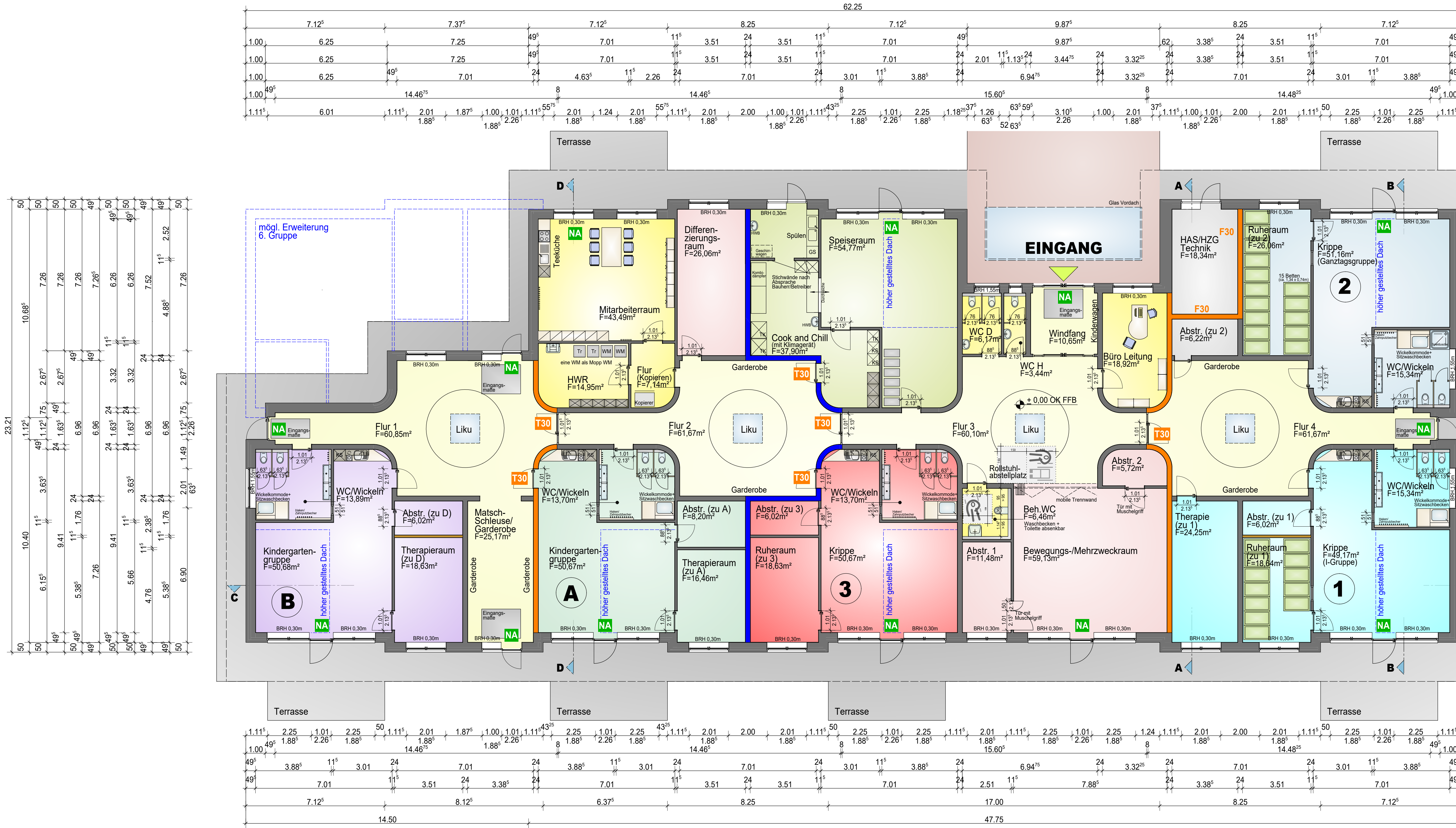
Grundriss Kindertagesstätte mit 5 Gruppen
